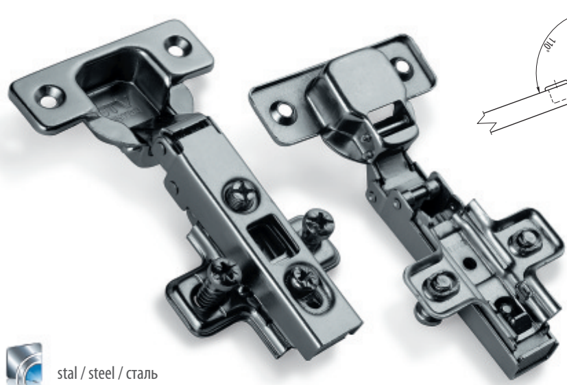
Regulacja pozioma Horizontal adjustment Регулировка по горизонтали
