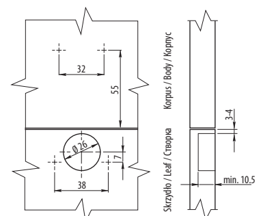
Wymiary montażowe / Mounting dimensions / Монтажные размеры
