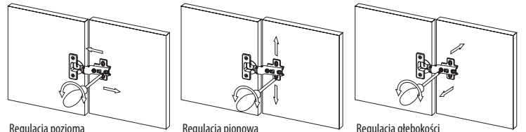
Regulacja pozioma Horizontal adjustment Регулировка по горизонтали
