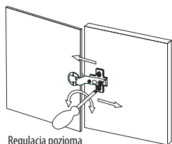
Regulacja pozioma Horizontal adjustment Регулировка по горизонтали
