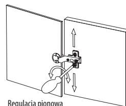
Regulacja pionowa Vertical adjustment Регулировка по вертикали
