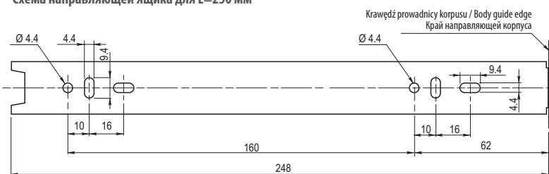
Schemat prowadnicy szuflady dla L=250 mm / Drawer guide scheme for L=250 mm Схема направляющей ящика для L=250 мм
