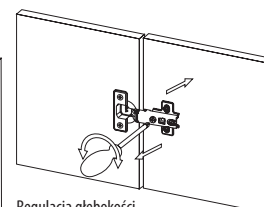
Regulacja głębokości Depth adjustment Регулировка глубины
