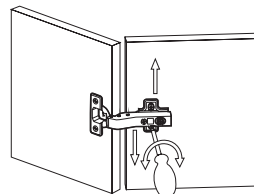
Regulacja pionowa Vertical adjustment Регулировка по вертикали
