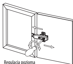
Regulacja pozioma Horizontal adjustment Регулировка по горизонтали
