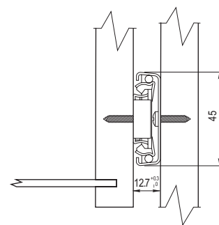
Pozycja mocowania prowadnic korpusu Fixing position of body guides Место крепления направляющих корпуса
