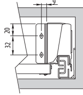
Wymiary montażowe mocowania tyłu Mounting dimensions of back fixing Монтажные размеры крепления задней части
