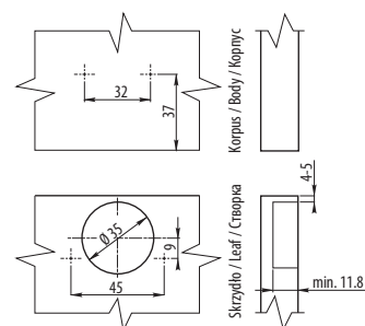
Wymiary montażowe / Mounting dimensions / Монтажные размеры
