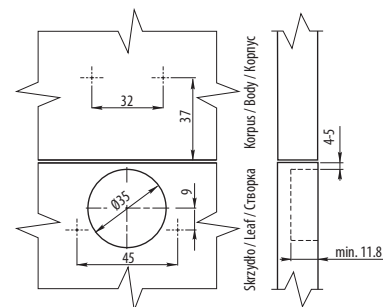
Wymiary montażowe / Mounting dimensions / Монтажные размеры
