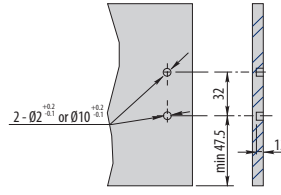
Wymiary montażowe frontu Mounting dimensions of front Монтажные размеры фасада
