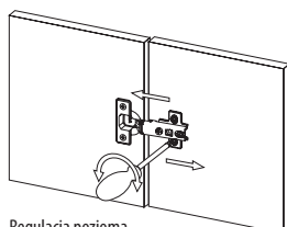
Regulacja pozioma Horizontal adjustment Регулировка по горизонтали
