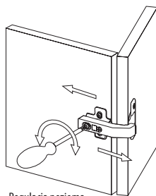
Regulacja pozioma Horizontal adjustment Регулировка по горизонтали
