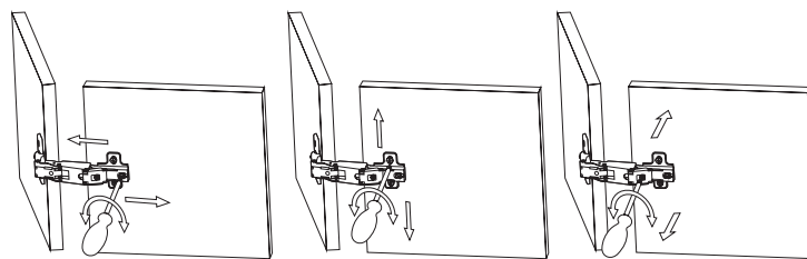
Regulacja pozioma Horizontal adjustment Регулировка по горизонтали
