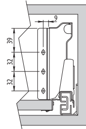
Wymiary montażowe mocowania tyłu Mounting dimensions of back fixing Монтажные размеры крепления задней части
