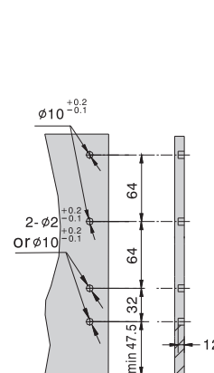
Wymiary montażowe frontu Mounting dimensions of front Монтажные размеры фасада
