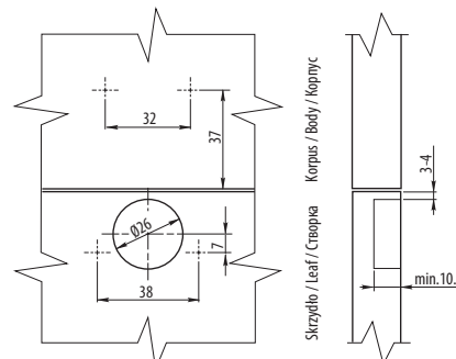
Drzwi otwarte / Door opened Открытые дверцы
