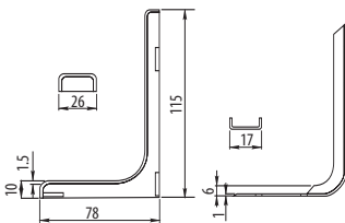
Oslona 12 Cover 12 Оболочка 12
