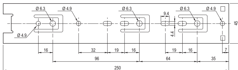
Schemat prowadnicy korpusu dla L=250 mm / Body guide scheme for L=250 mm Схема направляющей корпуса для L=250 мм
