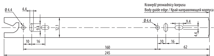
Schemat prowadnicy korpusu dla L=250 mm / Body guide scheme for L=250 mm Схема направляющей корпуса для L=250 мм
