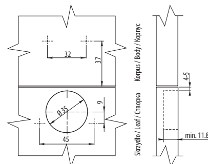
Wymiary montażowe / Mounting dimensions / Монтажные размеры
