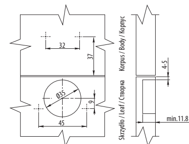
Wymiary montażowe / Mounting dimensions / Монтажные размеры
