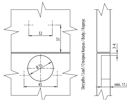
Wymiary montażowe / Mounting dimensions / Монтажные размеры
