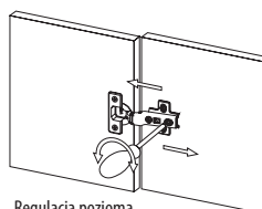
Regulacja pozioma Horizontal adjustment Регулировка по горизонтали
