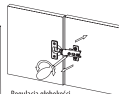
Regulacja głębokości Depth adjustment Регулировка глубины
