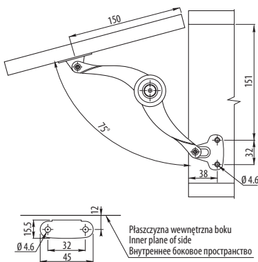
Drzwi nakładane 75° / Lift-off door 75° / Наружные дверцы 75°
