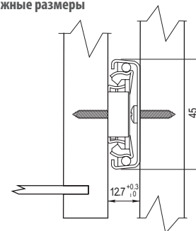
Wymiary montażowe / Mounting dimensions Монтажные размеры
