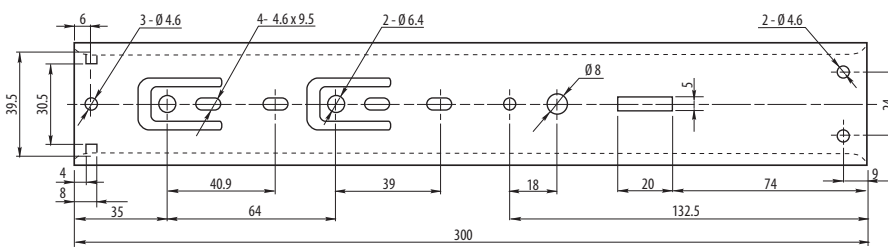
Schemat prowadnicy szuflady dla L=300 mm / Drawer guide scheme for L=300 mm Схема направляющей ящика для L=300 мм
