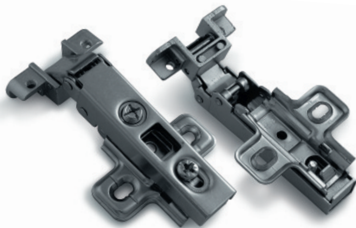
Regulacja pozioma Horizontal adjustment Регулировка по горизонтали
