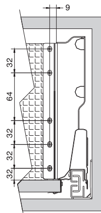
Wymiary montażowe mocowania tyłu Mounting dimensions of back fixing Монтажные размеры крепления задней части
