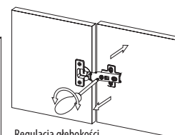
Regulacja głębokości Depth adjustment Регулировка глубины
