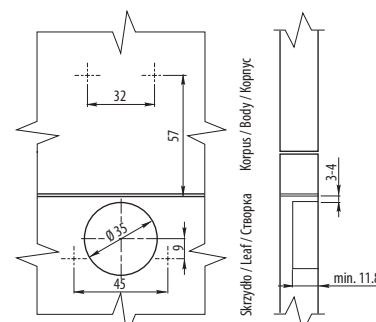
Wymiary montażowe / Mounting dimensions / Монтажные размеры
