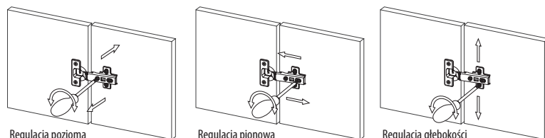
Regulacja pozioma Horizontal adjustment Регулировка по горизонтали
