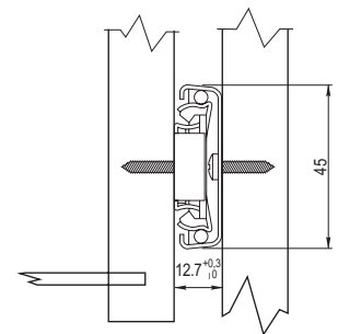
Wymiary montażowe / Mounting dimensions Монтажные размеры
