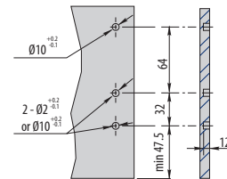
Wymiary montażowe frontu Mounting dimensions of front Монтажные размеры фасада
