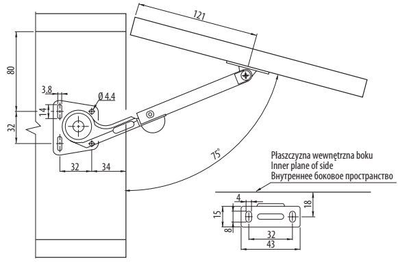
Drzwi nakładane 75° / Lift-off door 75° / Наружные дверцы 75°
